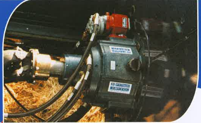
HPTO オイルクラッチ 自動調整HPTO オイルクラッチ
