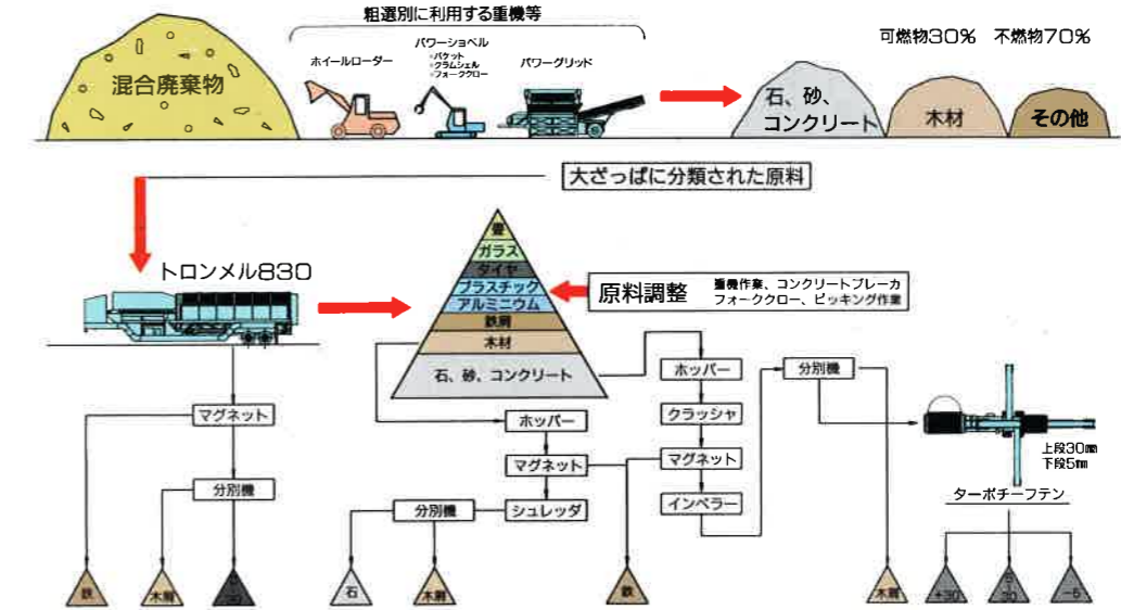
産業廃棄物処理システムフローシート 参考図
