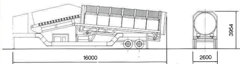
■外形寸法 MK830
