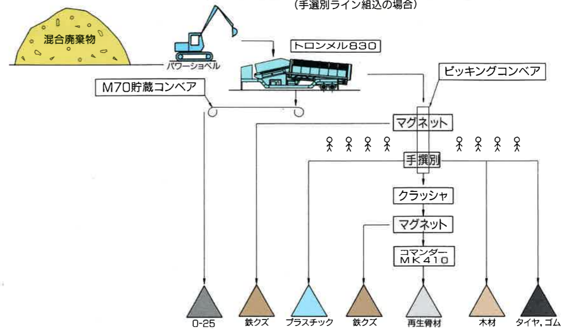
産業廃棄物処理ピッキングシステムフローシート 参考図 (手選別ライン組込の場合)
