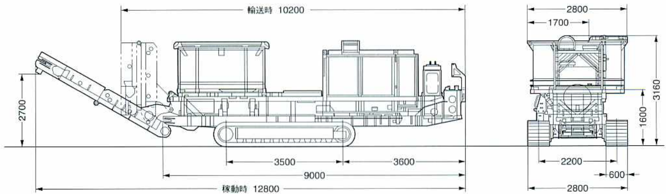
図、寸法はTG400ATX (単位mm)
